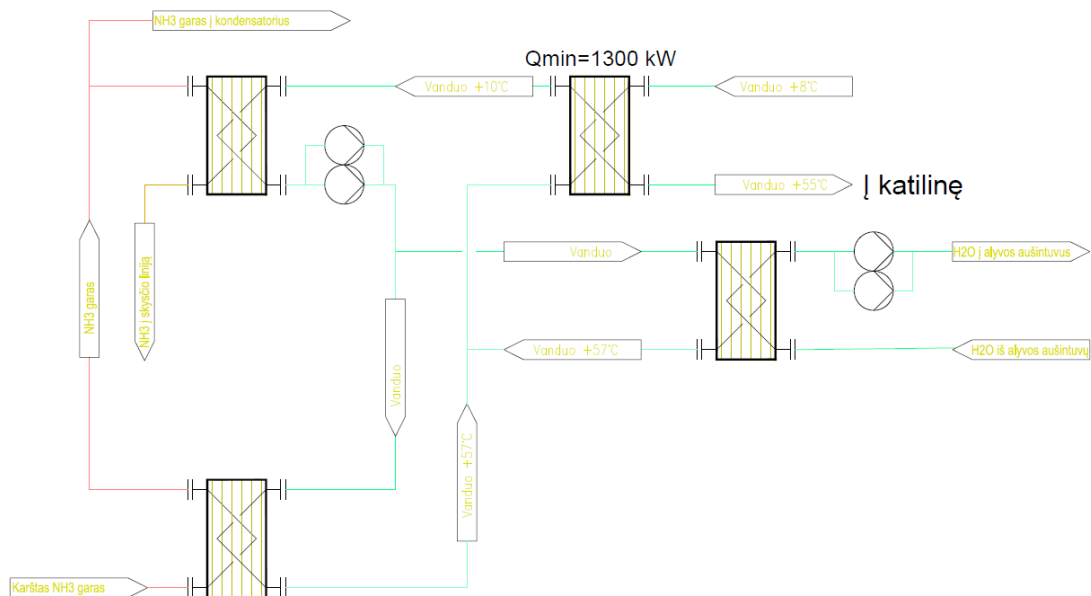
Pav. 3 Preliminari šilumos rekuperacijos schema
