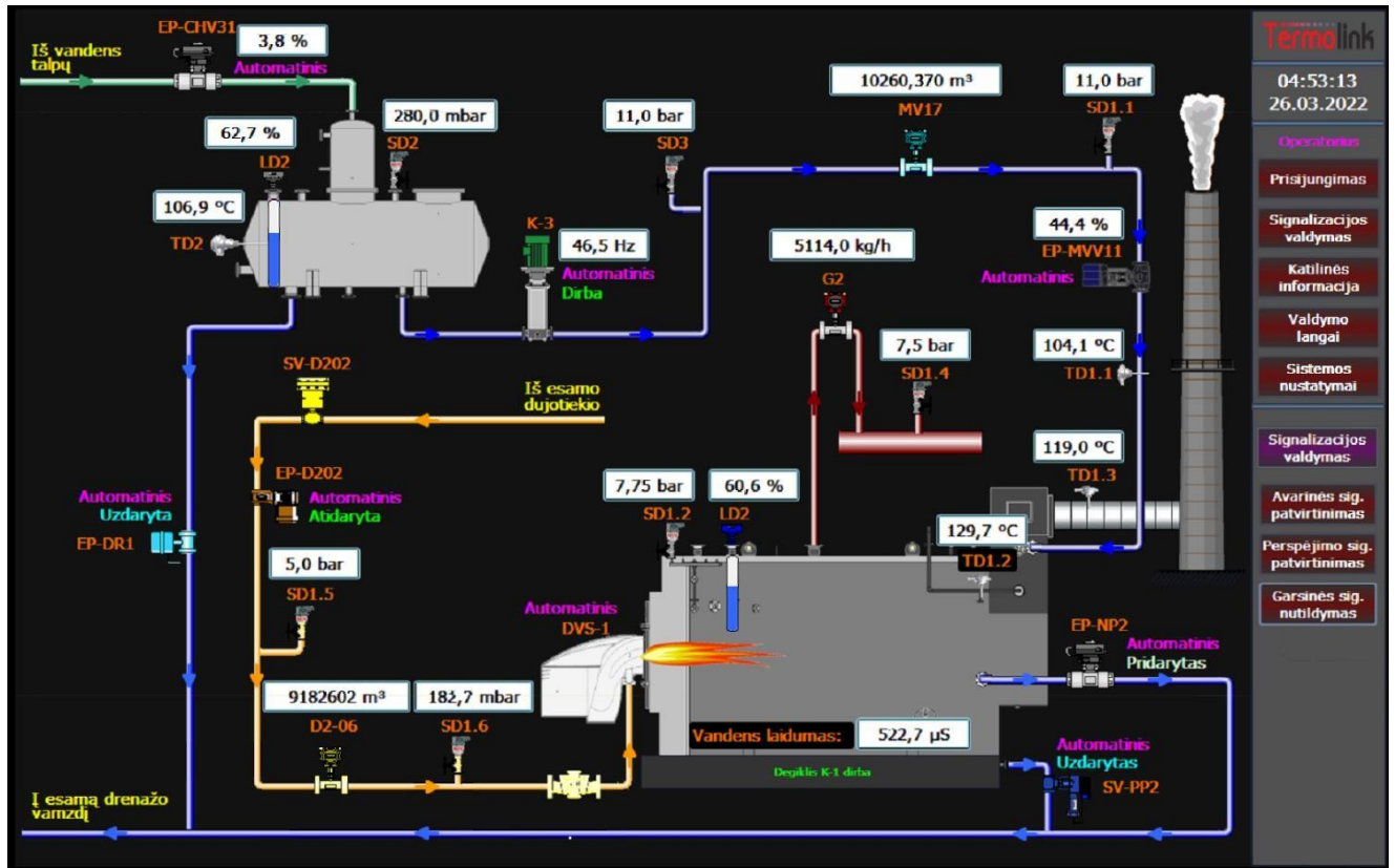
Pav. 2 Katilinės schema
