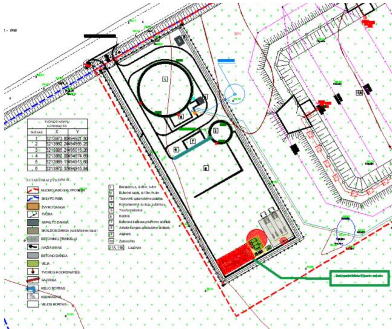
1 pav. Esamų ir planuojamų įrenginių / statinių planas
