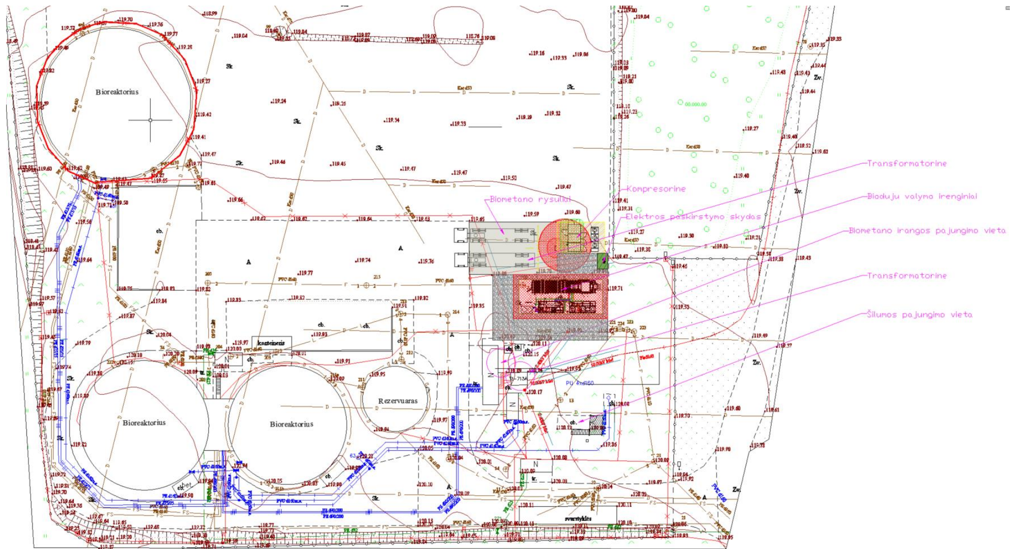
1 pav.: UAB SENERGITA ESAMŲ IR PLANUOJAMŲ ĮRENGINIŲ / STATINIŲ PLANAS
