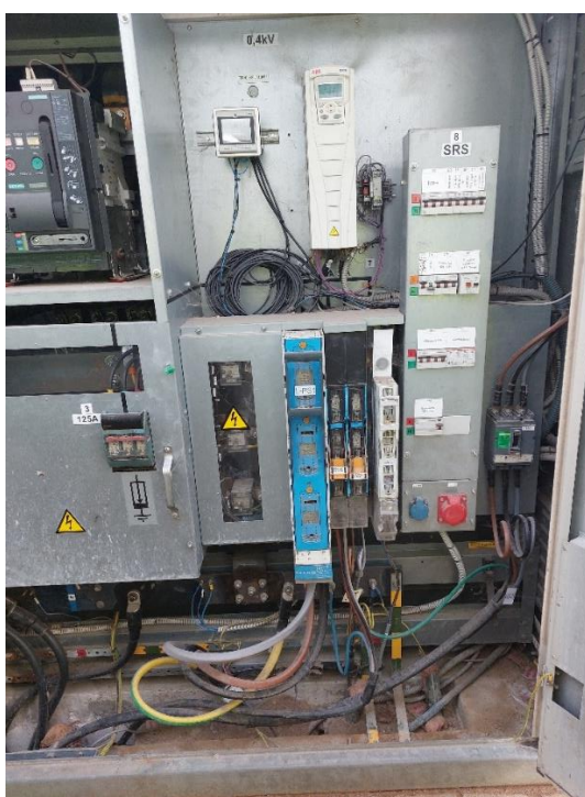
4 pav. Modulinės transformatorinės Nr. Tt-713A, 0,4kV dalies vaizdas
