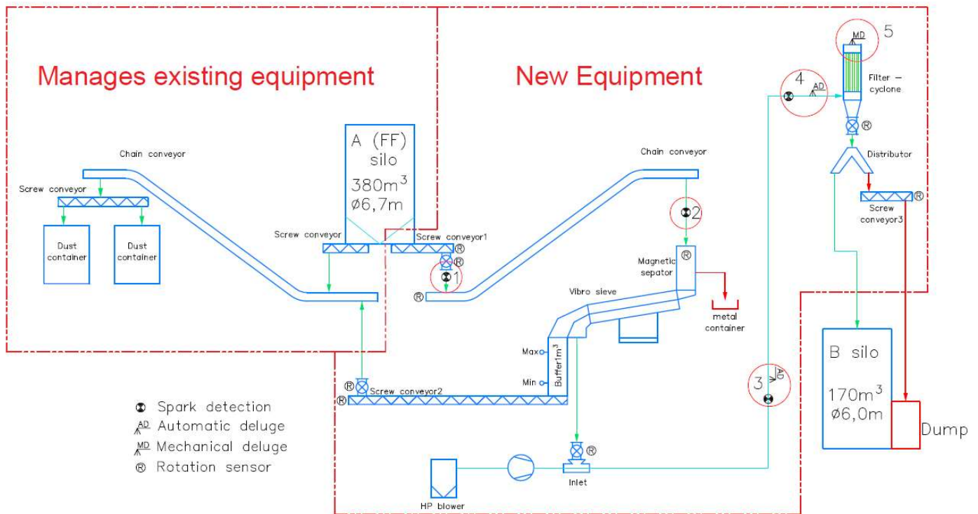
Paveikslas Nr. 12. Automatikos – valdymo sistemos schema
