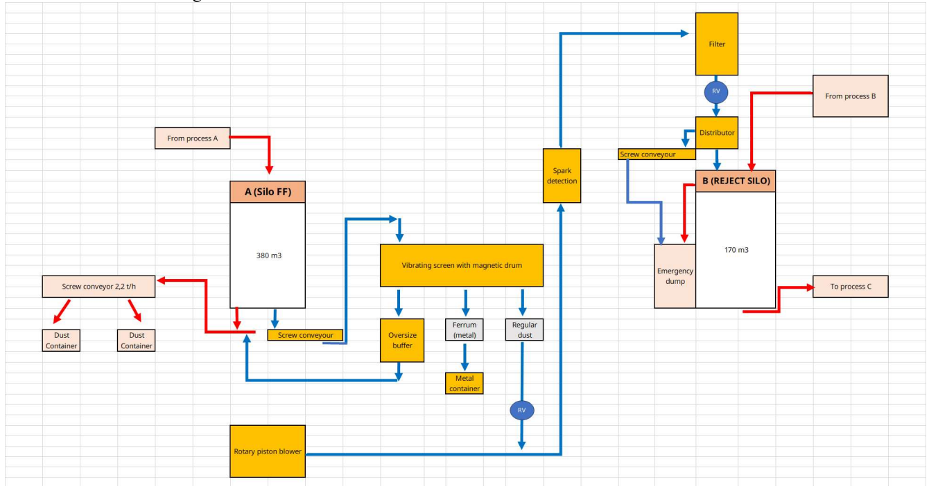
Paveikslas Nr. 2. Technolinė schema.
