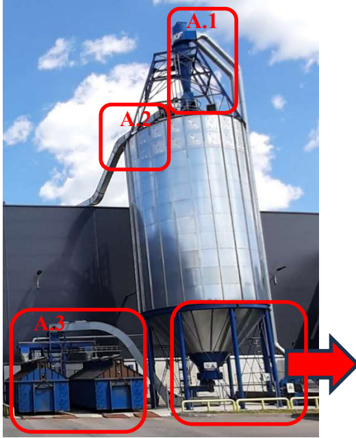
Paveikslas Nr. 4. Dulkių saugojimo sistema – silosas (380 m 3 /100t).
