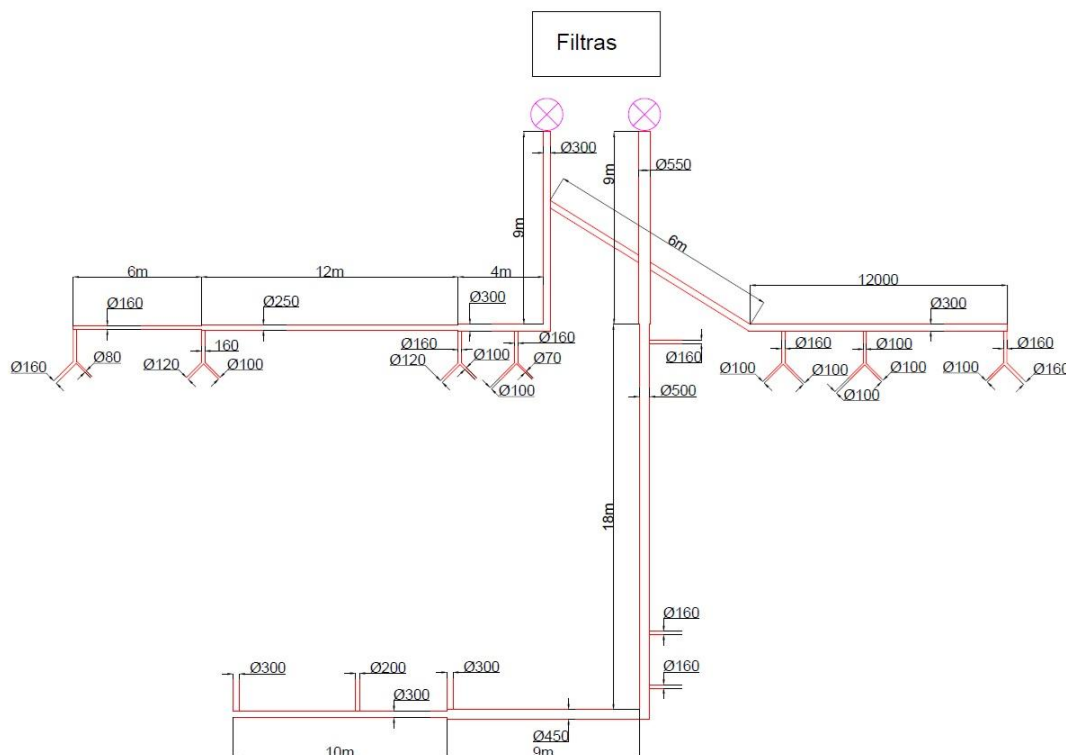
Paveikslas Nr. 3: Esamo vamzdyno schema
