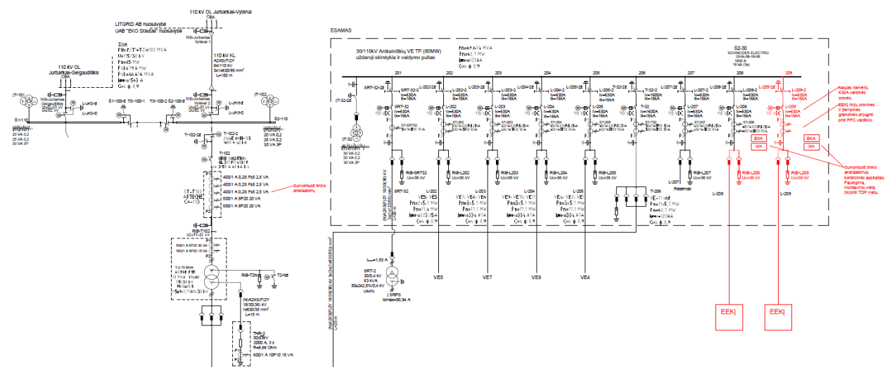
2 pav. Antkalniškių VE TP 110/30 kV principinė elektros schema
